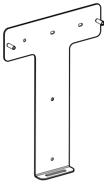
Befestigungswinkel × 1
